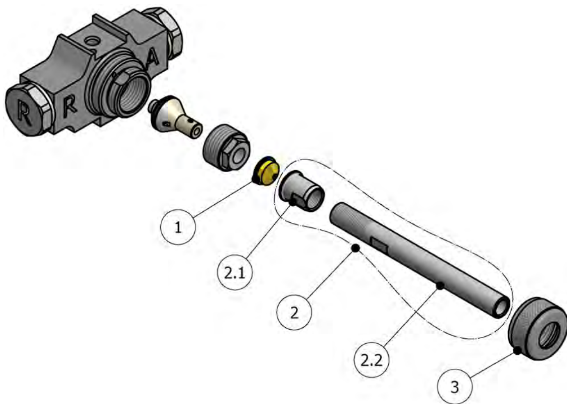
Figura 9. Ensamblaje para Colada (Opcional)
