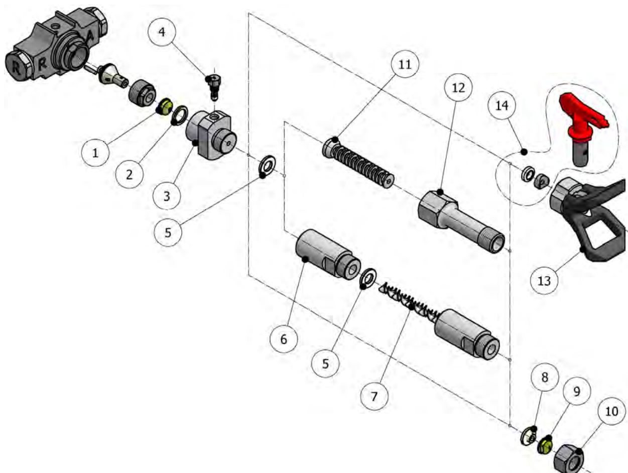
Figura 8. Ensamblajes Especiales de Proyección (Opcional)
