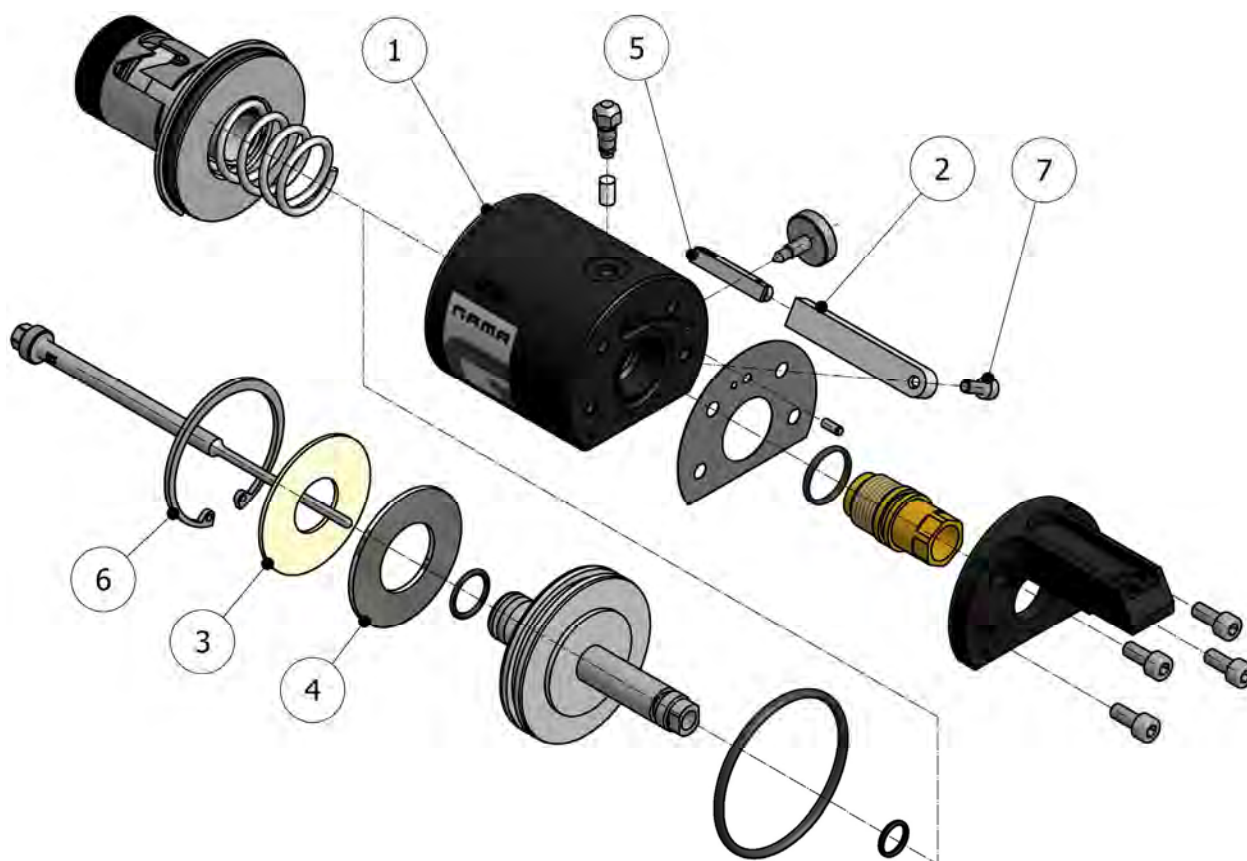
Figura 3. Ensamblaje Émbolo Magnético (Opcional), Pistola G-DI
