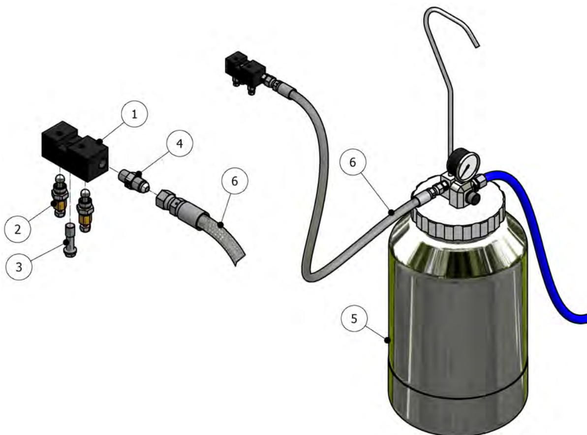
Figura 11. Kit de Limpieza (Opcional) KT-00072
