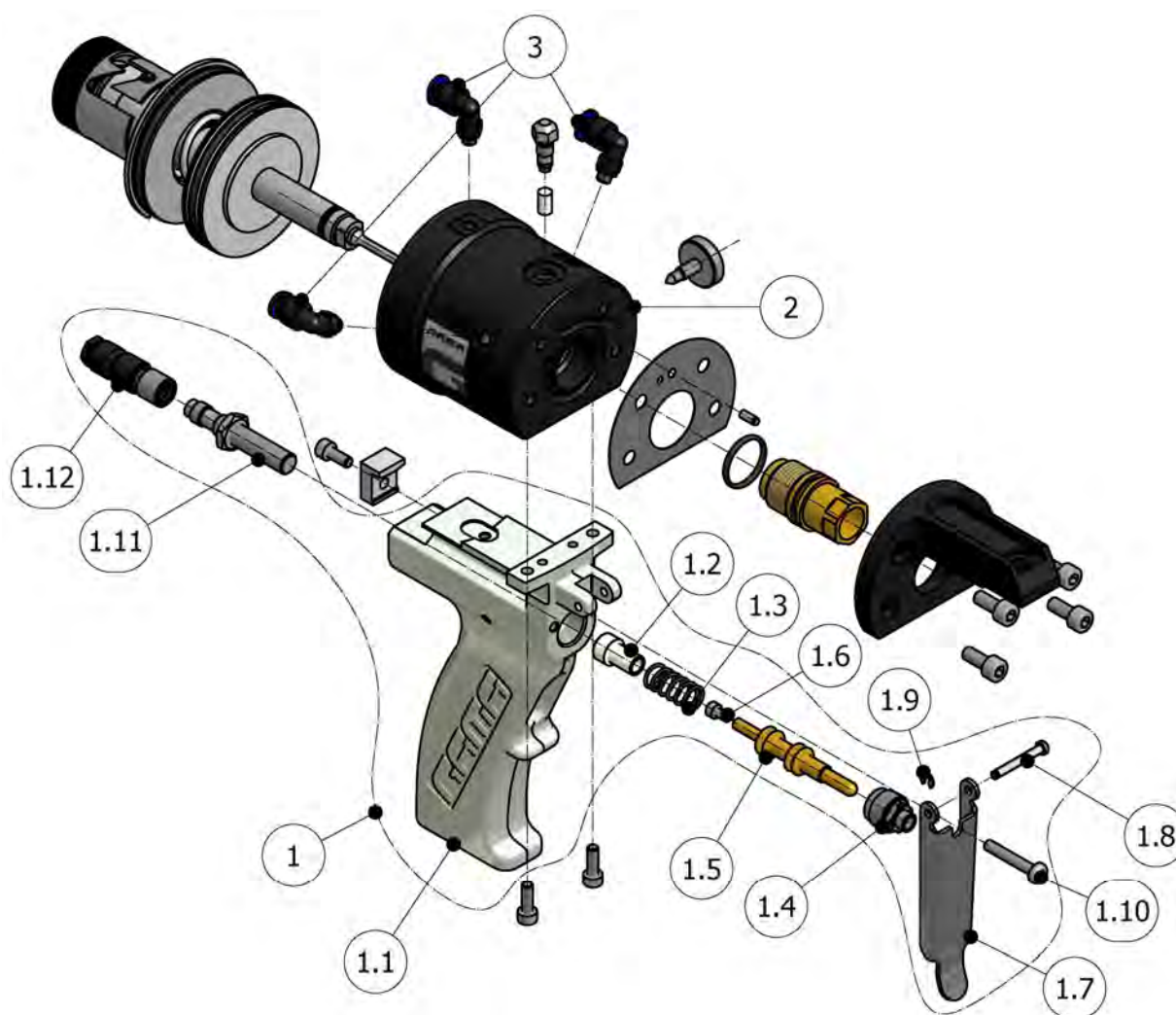
Figura 4. Ensamblaje Temporizador (Opcional), Pistola G-DI
