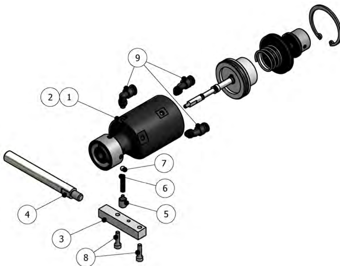
Figura 7. Ensamblaje para Versión Auto (OPCIONAL)
