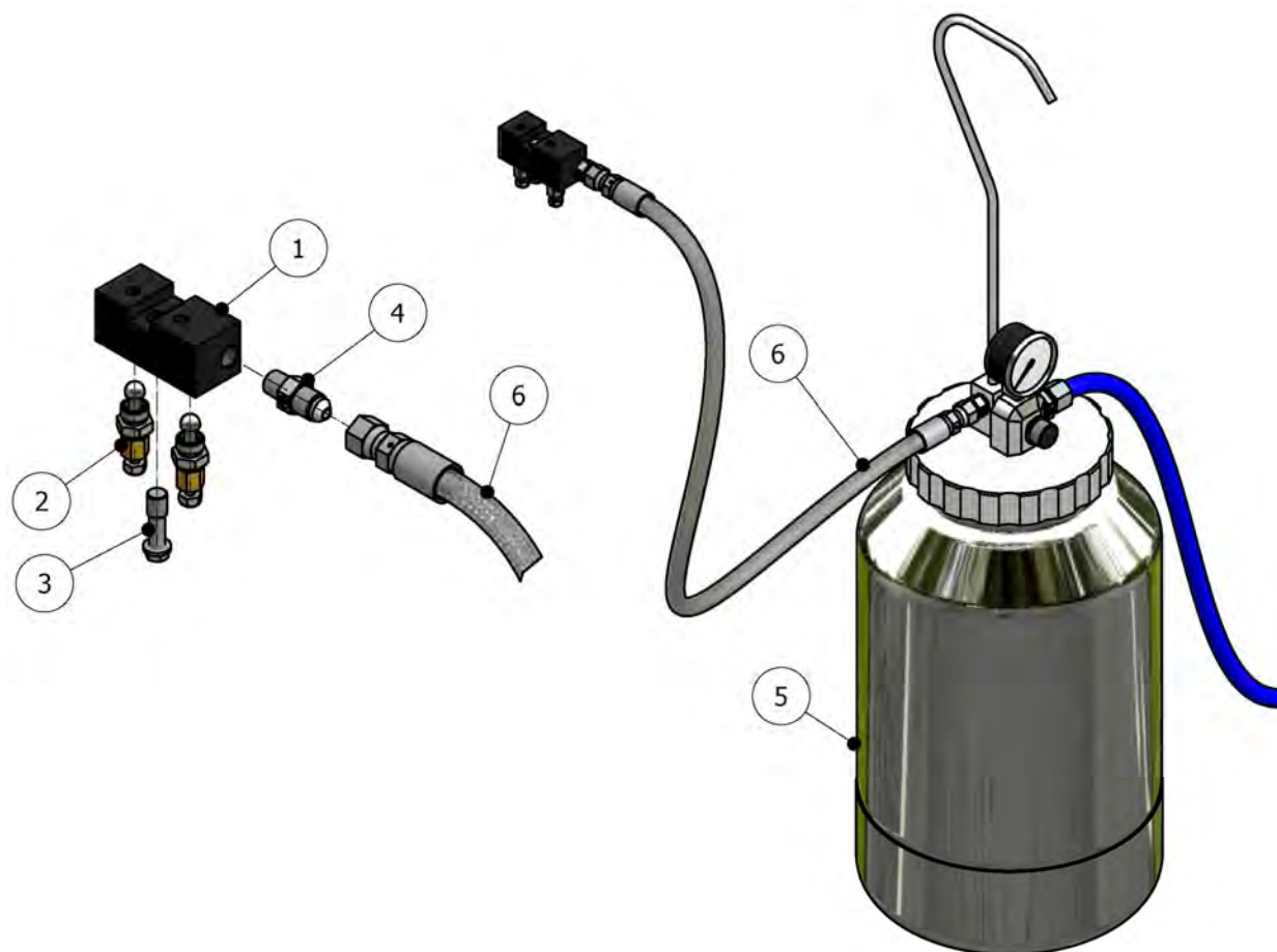
Figura 13. Kit de Limpieza (OPCIONAL) KT-00072
