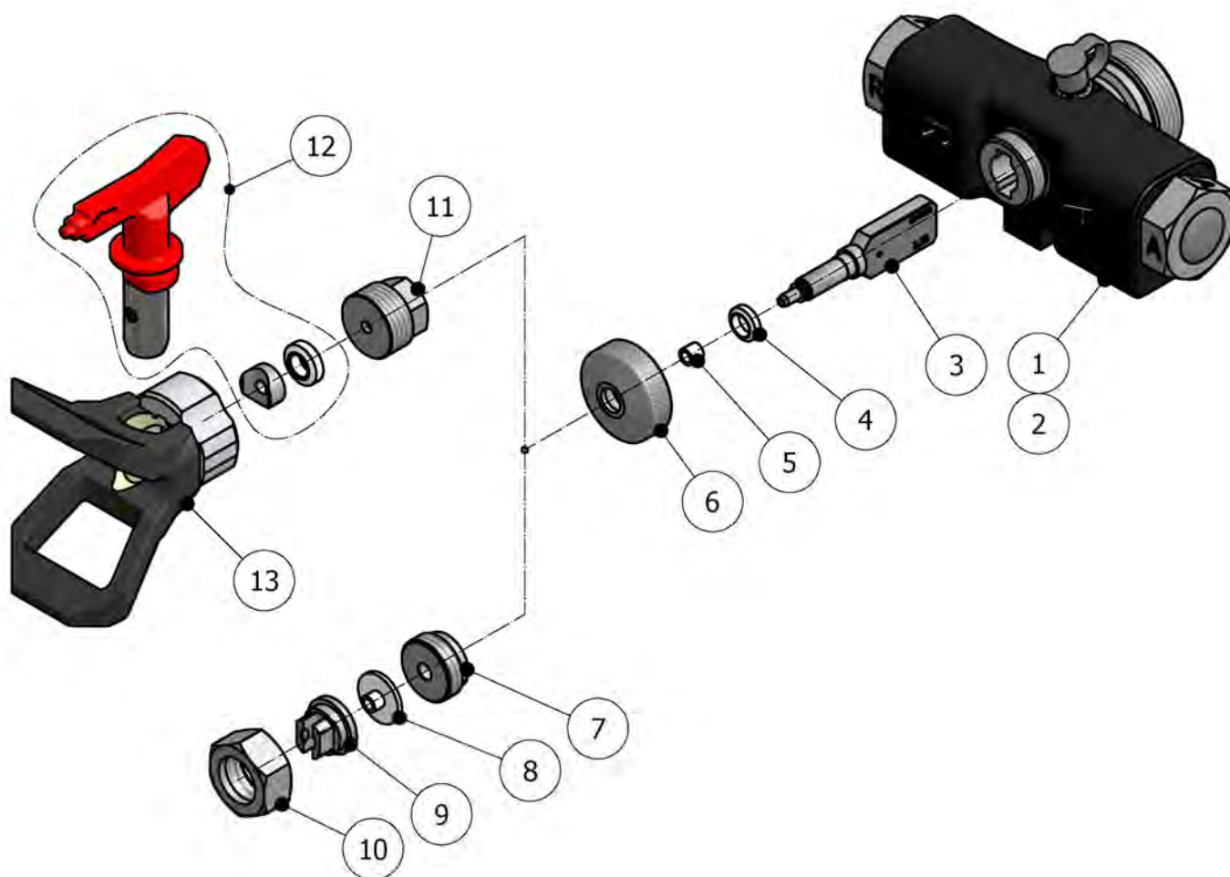
Figura 9. Ensamblaje Abanico Plano
